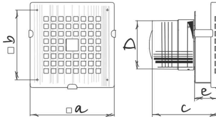
Dimensiones [mm]
